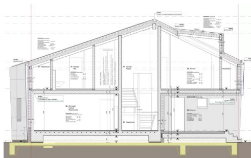
Haus am See I, Schnitt
